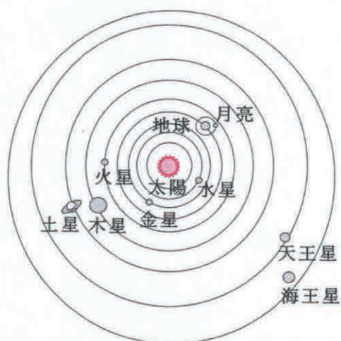
八大行星公轉軌道(圖2-11)
